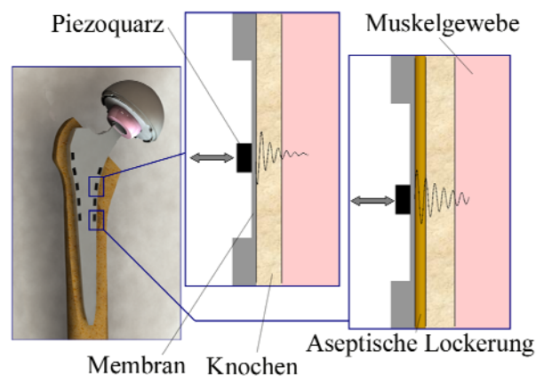
Abb. 1: Prinzip des Sensorsystems für die Diagnose einer aseptischen Lockerung in Hüftendoprothesen
