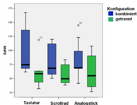
Abb. 3: Dargestellt sind die Boxplots für den HRV-Parameter SdNN, jeweils für die einzelnen Eingabemodule (Tastatur, Scrollrad, Analogstick). Zwischen der kombinierten und getrennten Konfiguration des tastaturbasierten MIS bestehen statistisch signifikante Unterschiede ( p < 0,05 ; Mann-Whitney-U Test).
