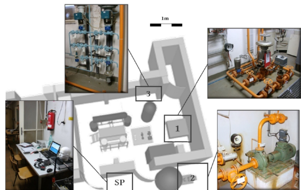
Abb. 1: Die Belastungsbedingungen wurden in einem industriellen Wartungsszenario nachgebildet. Die Aufgaben bestanden u.a. in der visuellen Inspektion sowie dem Öffnen und Schließen von Ventilen und Gehäusen.
